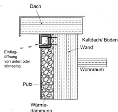
Hinterdämmter Einbaustein
