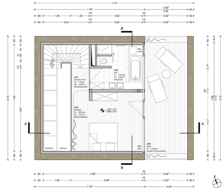
Grundriss 2. OG M 1:50
