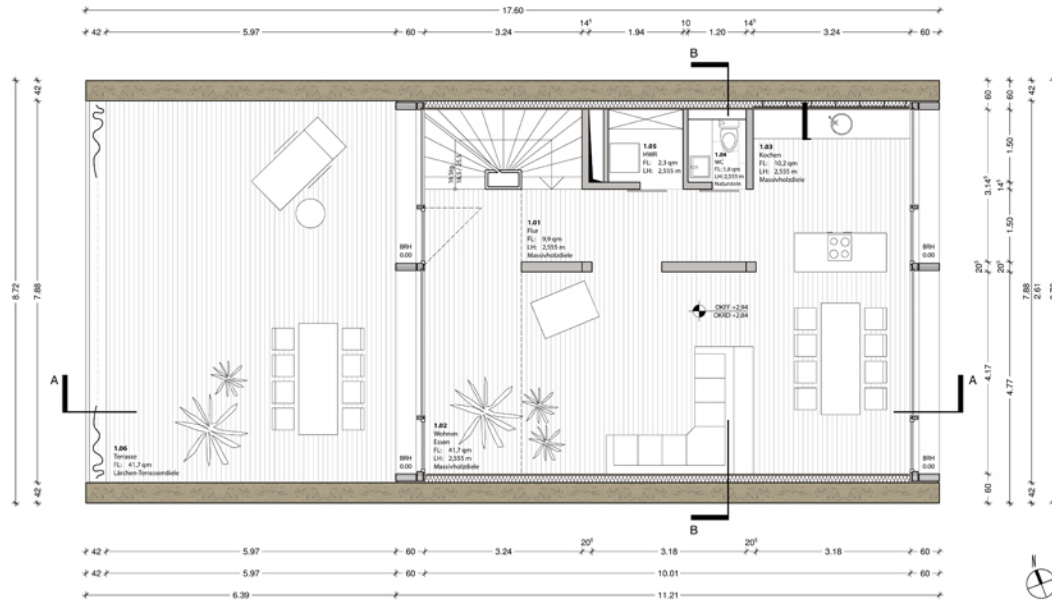
Grundriss 1. OG M 1:50
