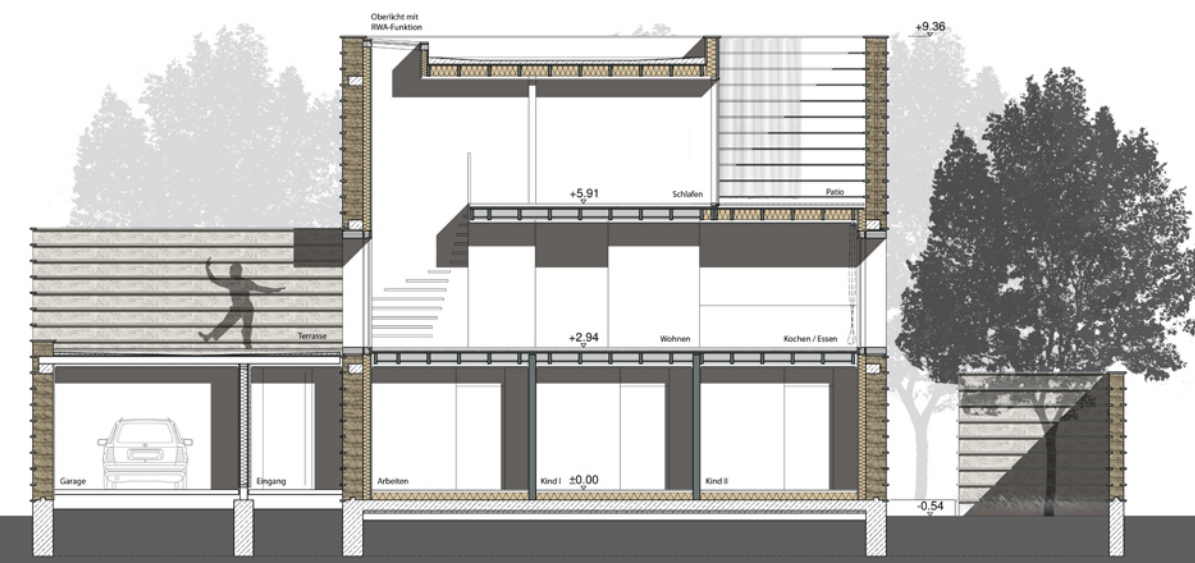
Schnitt A-A M 1:50
